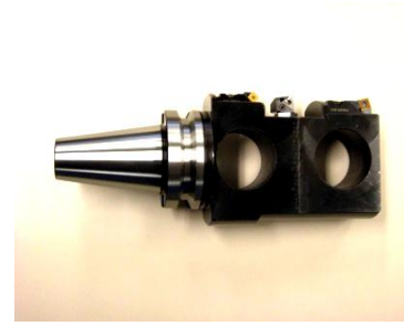
ボーリングバー(軽量化)
